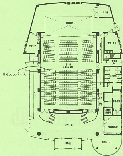
1階平面図
