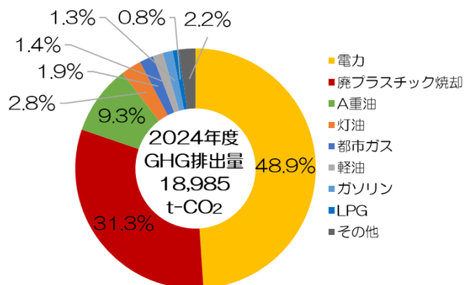
図5 燃料種別温室効果ガス構成比
