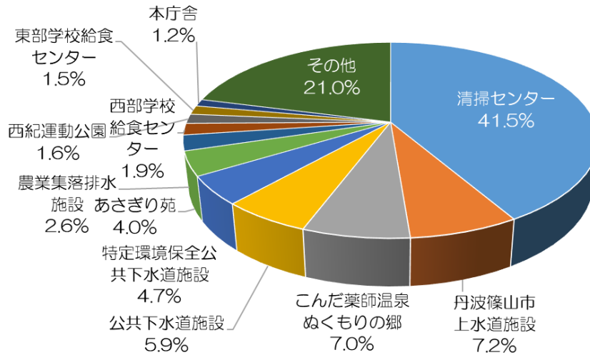
図 6 施設別温室効果ガス排出量の構成比
