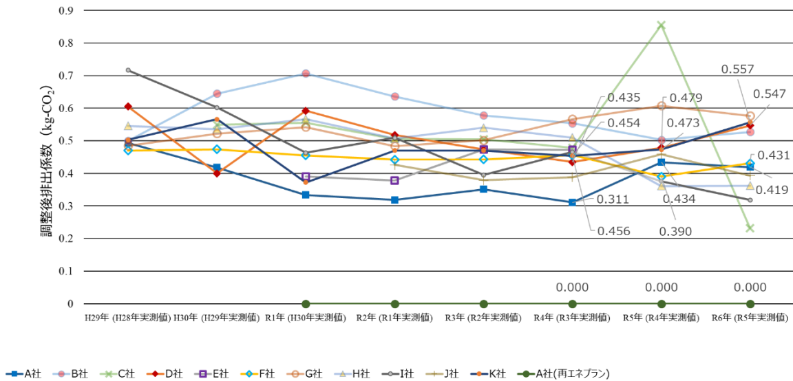
図8 市関連施設の平均排出係数の推移
