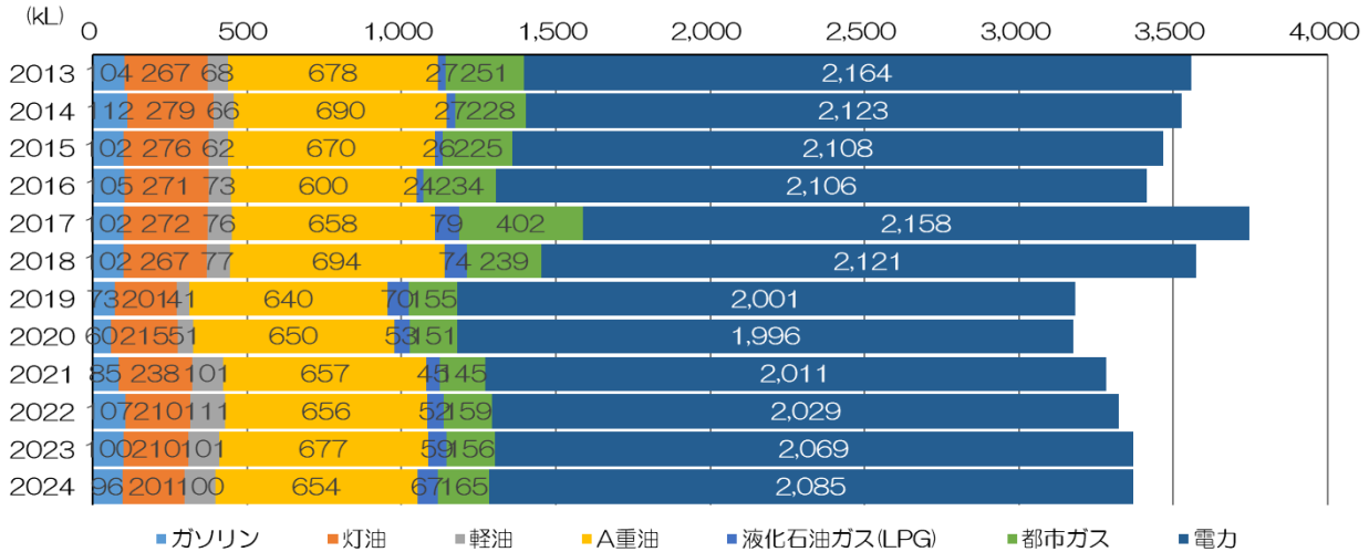
図3 燃料別エネルギー消費量の推移（原油換算）
