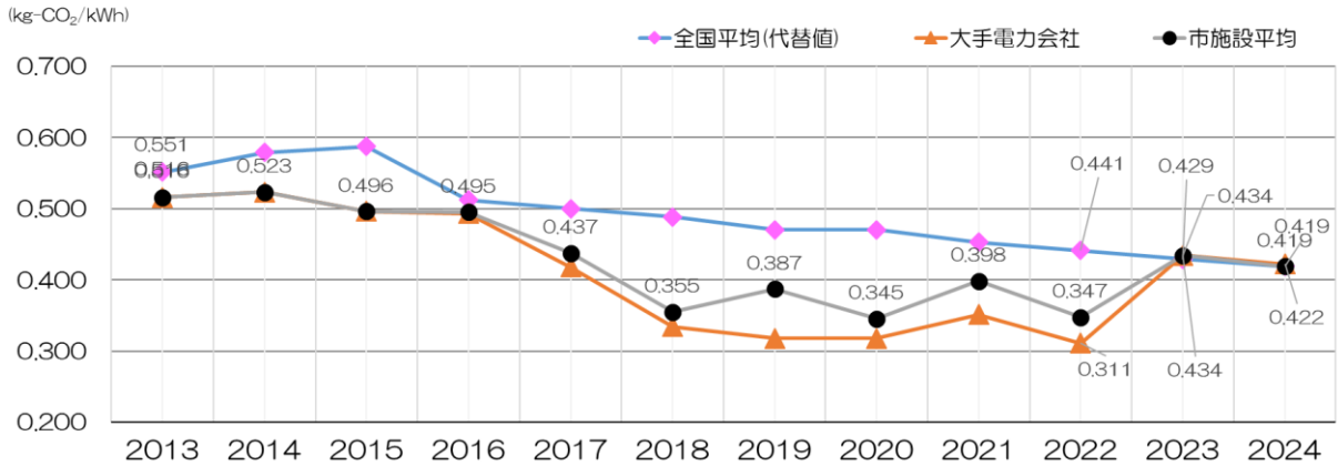
図8 市関連施設の平均排出係数の推移
