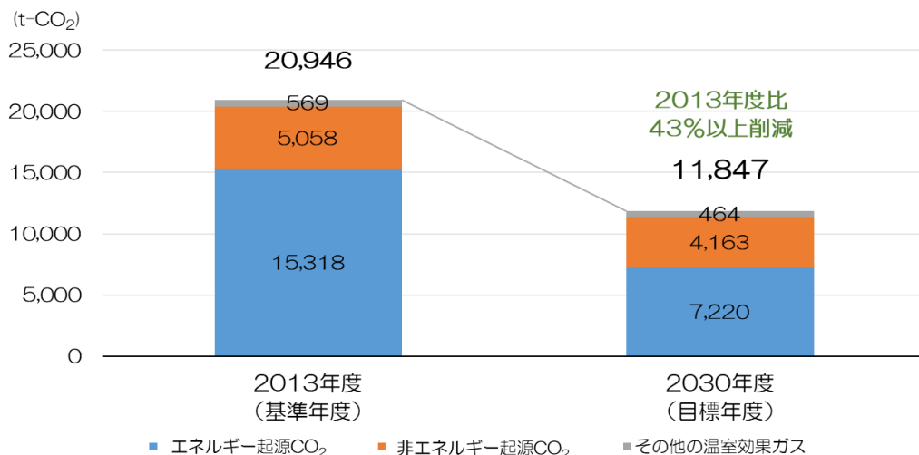
図1 温室効果ガス排出量の削減目標
