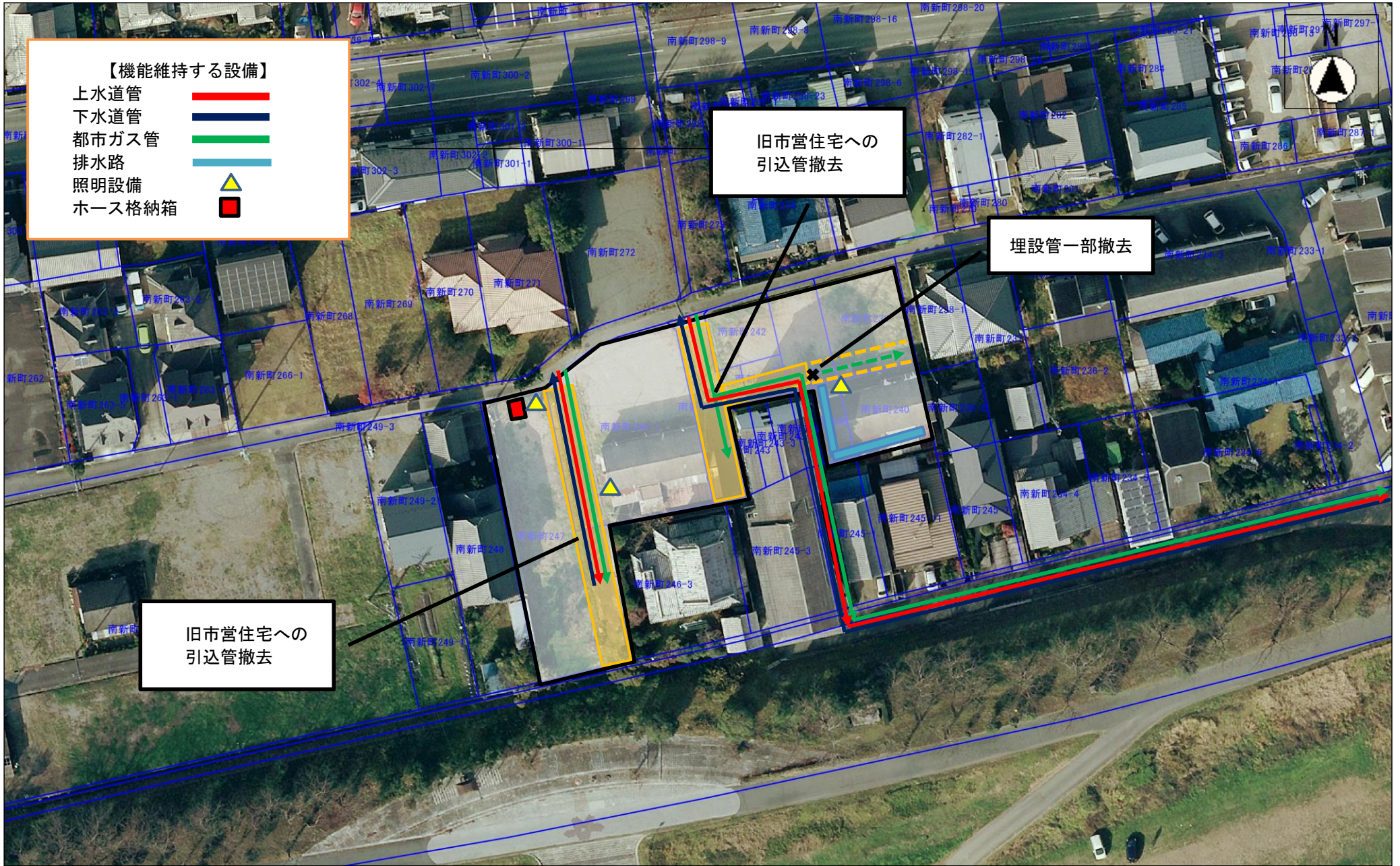
南新町市有地売却に係る機能維持設備等配置図
